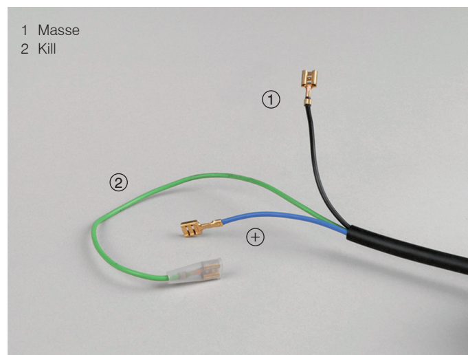
Kabelast zum Motor
