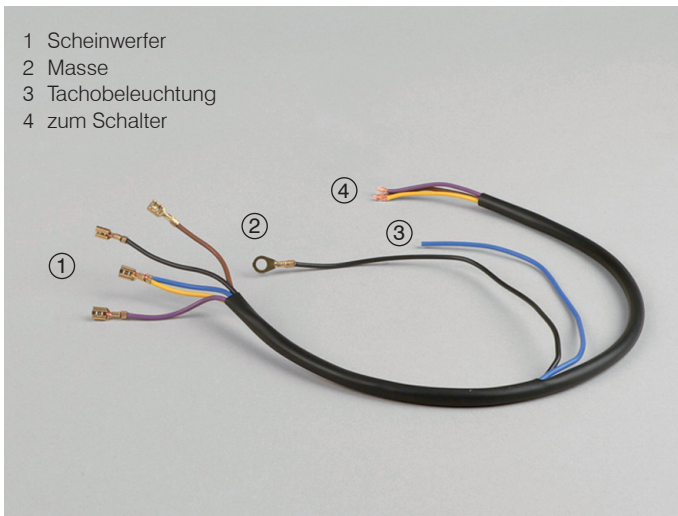
Kabelast im Lenker
