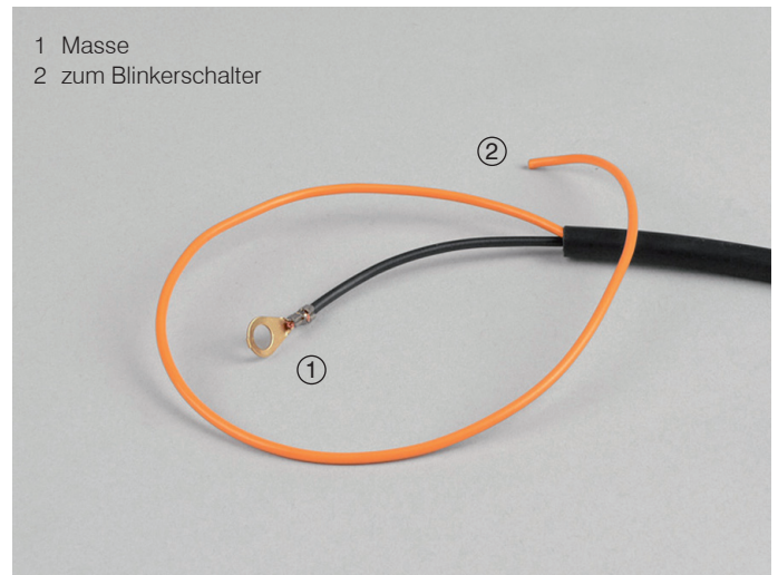
Kabelast im Lenker
