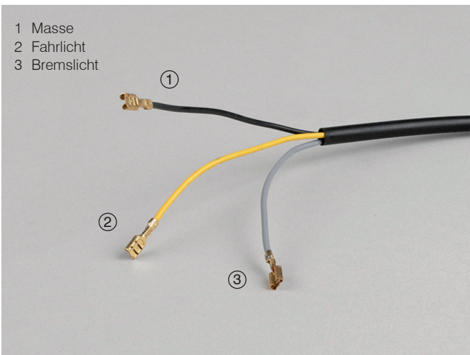
Kabelast zum Rücklicht
