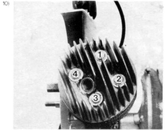
Schrauben (1-4) lösen (SW 11). Zylinderkopf abnehmen (Keine Dichtung).
