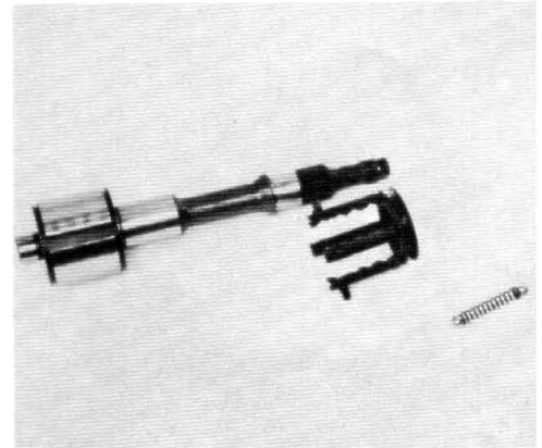
Schaltkreuz abziehen. (Mit der Hand zuhalten, daß die 2 Kugeln und die Feder nicht wegspringen).
