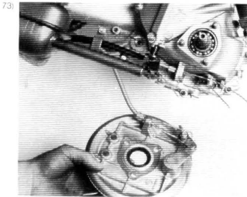
Bremsankerplatte abnehmen. Bremszug nicht lösen.
