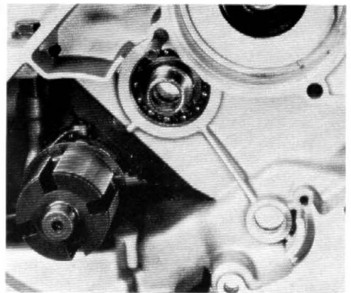
Antriebswelle einsetzen. Schaltsteine in Schaltring einführen
