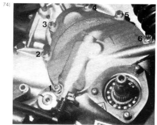
Schrauben (1-6) abschrauben (SW 10). Kupplungsdeckel mit Papierdichtung abnehmen.
