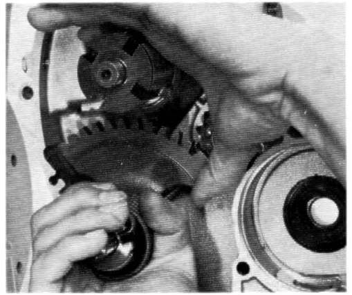
Kickstartersegment mit Feder abziehen. Kickstarterritzel mit Feder und Scheibe abnehmen.
