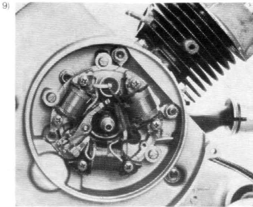
Schrauben (1-3) lösen. Grundplatte abnehmen.
