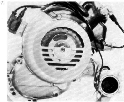
Lüfterdeckel abschrauben.
