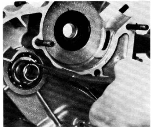
Kupplungswelle mit Seegerring sichern.
