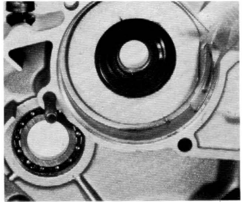
Simmerring montieren. Dichtlippen zur Kurbelwellenseite.
