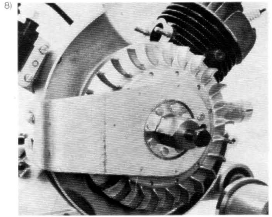
Rotor mit Halteschlüssel Nr. T 032 972 abziehen. Ab Baujahr 1979 mit Schlüssel Nr. T 048 564.
