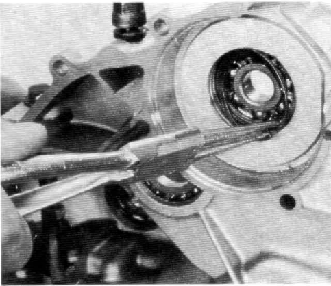
Seegerring einfedern.
