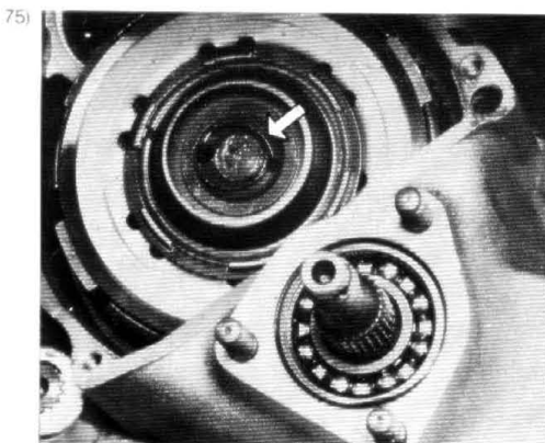
Kupplungsdruckplatte herausnehmen (nur durch Feder gehalten) (s. Pfeil).
