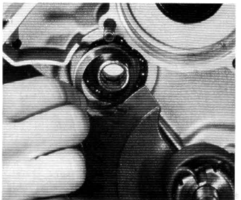
Schulterzscheibe montieren.
