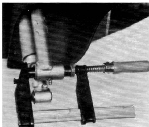
Nadellager einziehen.
