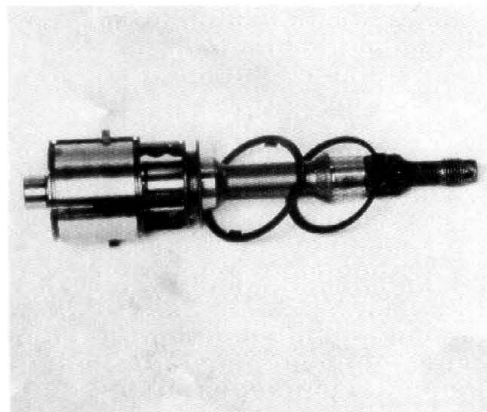
Beim Schaltkreuz auswechseln. Seegerring und Schulterring entfernen!
