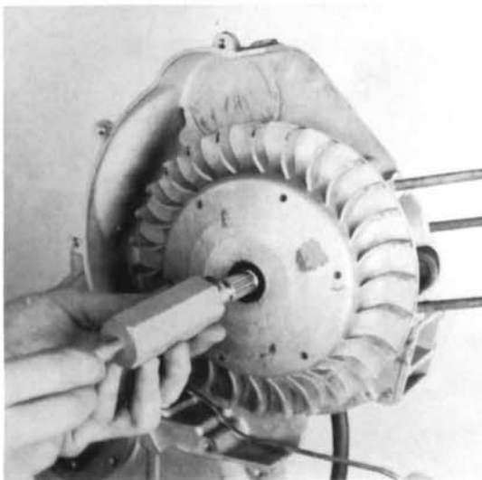
21) Polrad 19.1.20056 abziehen.
