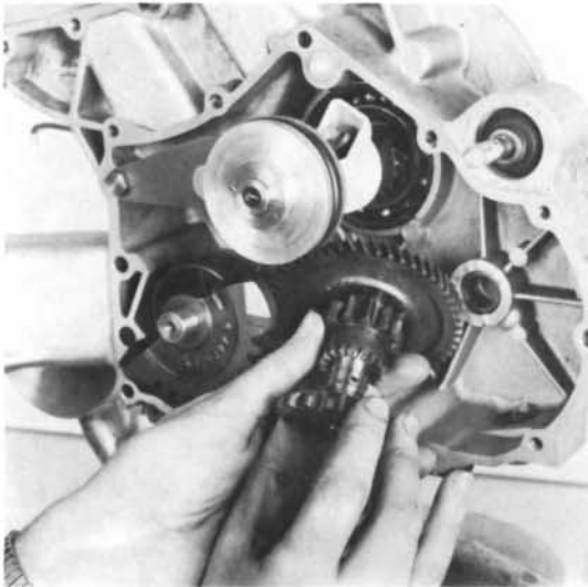
33) Vorgelegezahnrad herausziehen.
