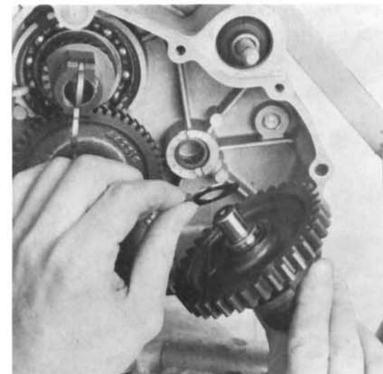
11) Scheibe montieren, Hinterachswelle einsetzen.
