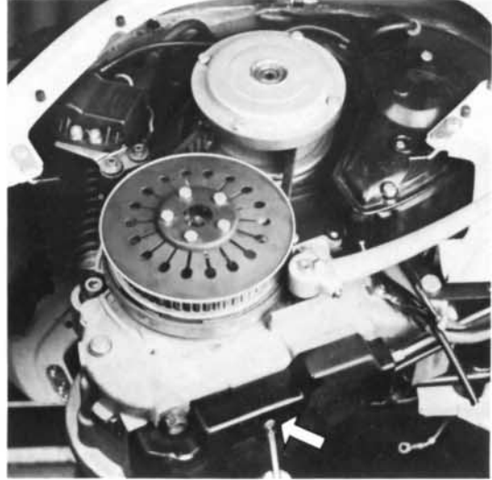
4) Abdeckkappe abschrauben.
