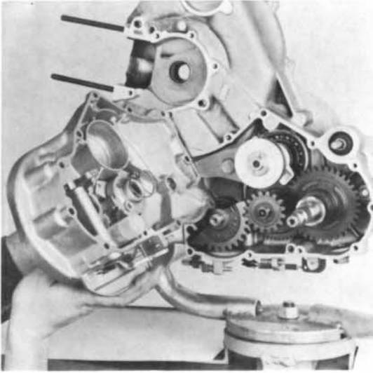
31) Gehäusehälfte.
