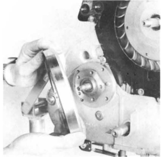
20) Kupplungstrommel abnehmen.
