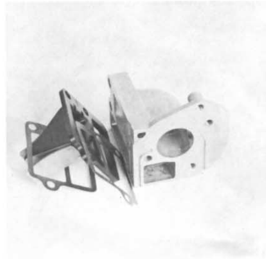
33) Membraneinlaßsteuerung mit Dichtung und Ansaugstutzen montieren. 3 Schrauben (SW 10) 6-8 Nm.
