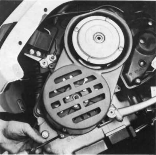
3) Gehäuseabdeckung abschrauben.
