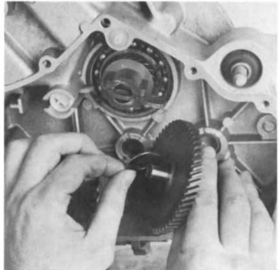
9) Anlaufscheibe auf Vorgelege montieren, Vorgelege einsetzen.
