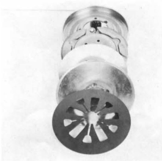
28) Kupplungskorb montieren. 4 Schrauben (SW 10) 8-10 Nm.
