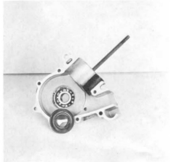
21) Gehäusehälften auf ca. 80 Grad erwärmen. Lager mit passendem Dorn einbauen. Seegerring einfedern. Wellendichtung montieren.
