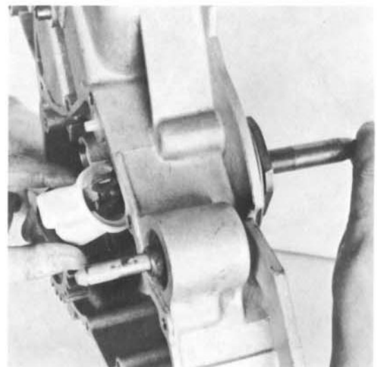
36) Steuerwelle herausziehen.
