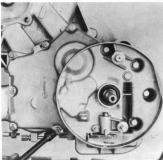
29) 11 Schrauben (SW 10) lösen.
