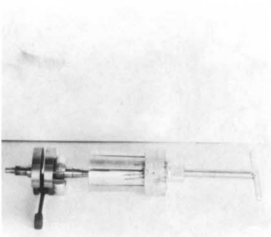
20) Lagerinnenring der Kurbelwelle (Lichtmaschinen- seite) abziehen. Werkzeug N. T 0014489.
