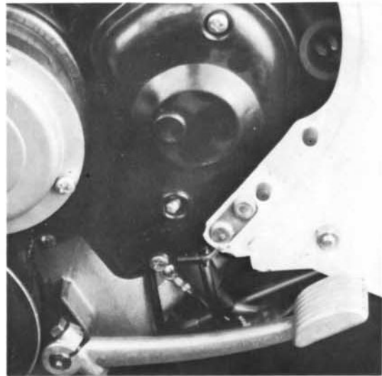
6) Schraube vom Kickstarter lösen (SW 14). Kickstarter abnehmen.
