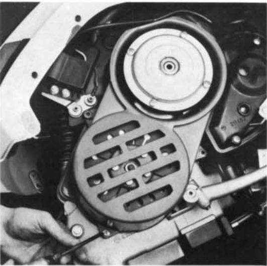
3) Gehäuseabdeckung abschrauben.
