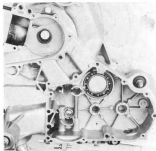
42) Lager und Nadellager mit passendem Dorn herausschlagen.
