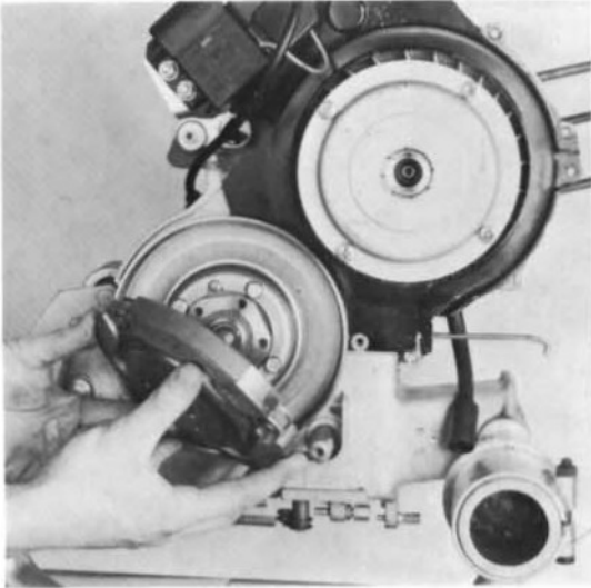
15) Kupplung abnehmen.
