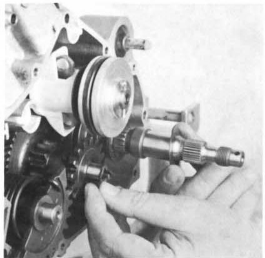
15) Anlaufscheibe einsetzen.
