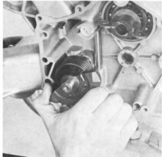
7) Kickstartersegment mit Welle einführen. Hierbei muß die Feder von Hand vorgespannt werden.
