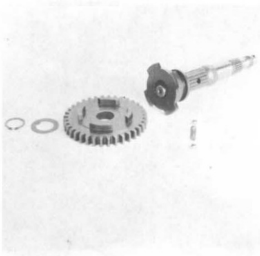
10) Seegerring und Schulterring entfernen. Zahnrad abziehen. Schiebemuffe abziehen. Mit der Hand zuhalten, damit die 2 Kugeln und die Feder nicht wegspringen können.
