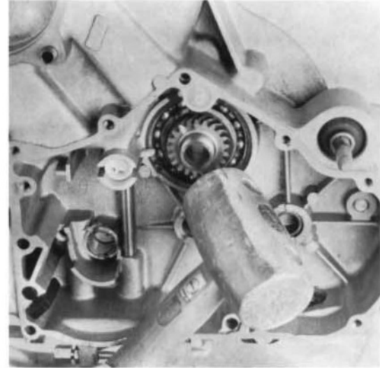
40) Zahnrad und Freilauf durch leichtes Klopfen auf dem Zahnrad nachhelfen.
