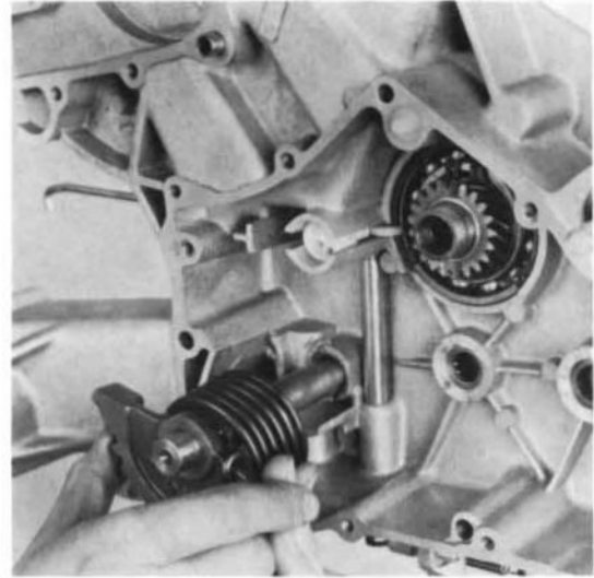
38) Kickstartersegment samt Feder aus dem Gehäuse herausziehen.
