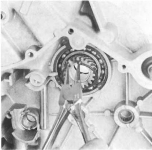
39) Sicherungsring entfernen.
